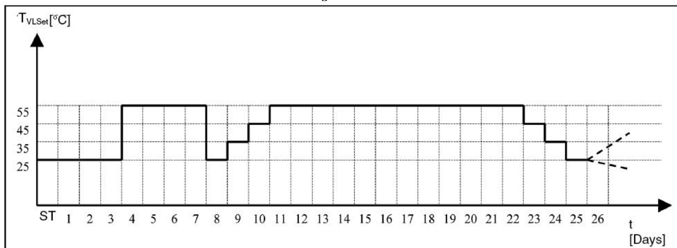
Zeitprofil für Schritt 1+2
