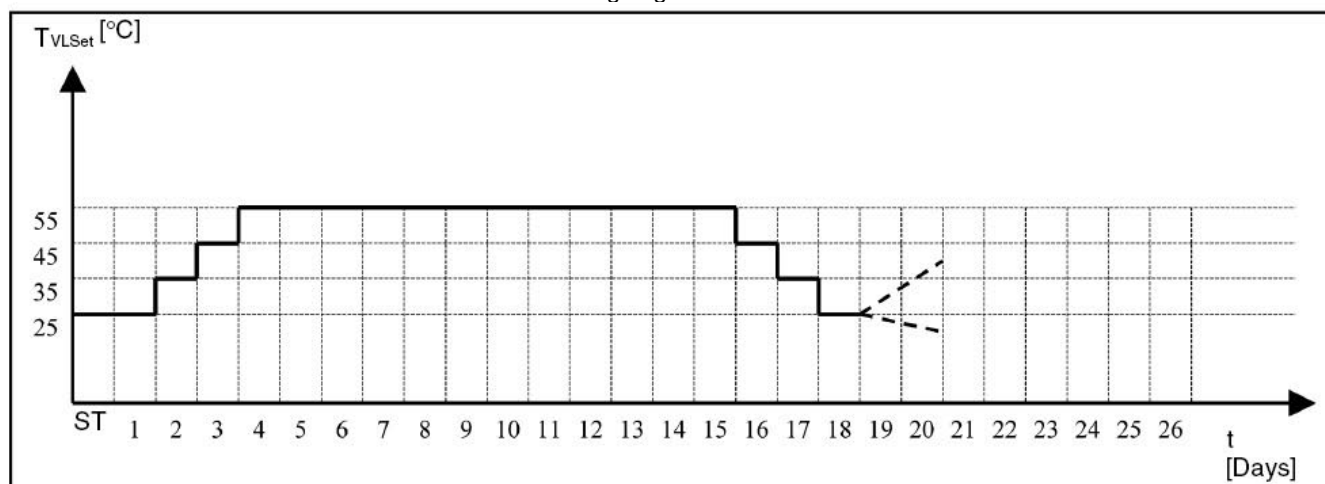
Zeitprofil für Fußbodenaushärtung
