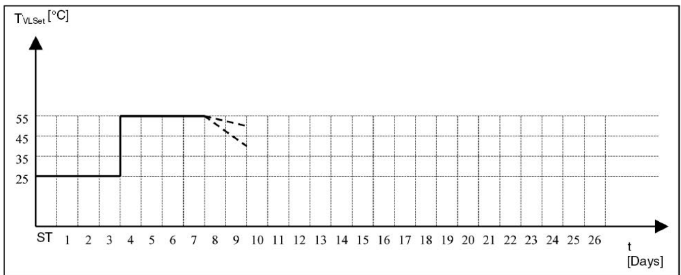
Zeitprofil für Austrocknung
