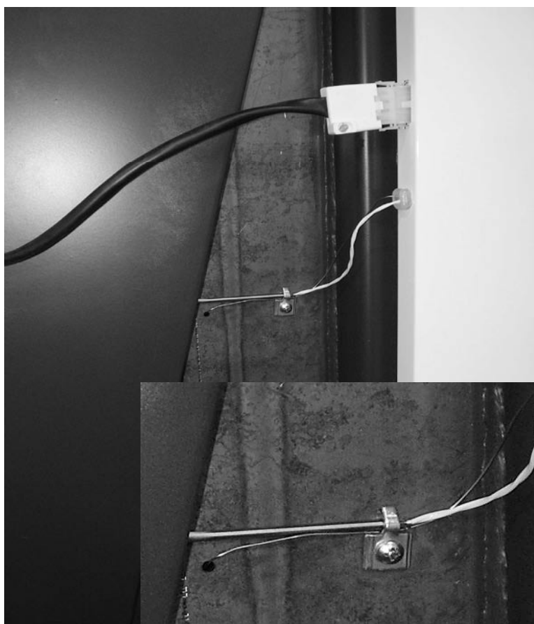
Angelegter Abgassensor am Kesselrauchabzug ( CxxS, DCxxS, DCxxR, DCxxSX, DCxxGS ), zugegeben zum Thermostatsensor ursprünglicher elektromechanischer Kesselregelung !!! Dieser Sensor muss mit Isolierung gedeckt werden !!!
